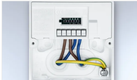
Grosser Anschlussraum
