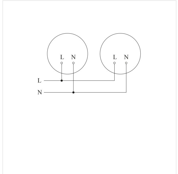
Schema elettrico Master-Master Bluetooth collegamento in rete
