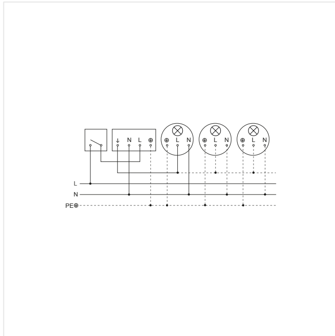
Schaltplan Leuchte mit vorhandenem Nullleiter
