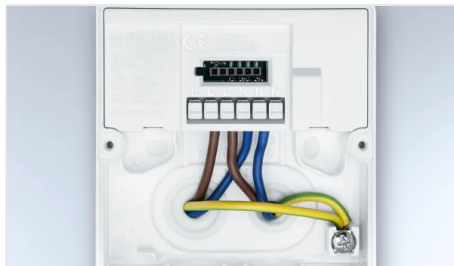
Grosser Anschlussraum
