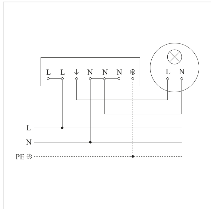
Schaltplan
