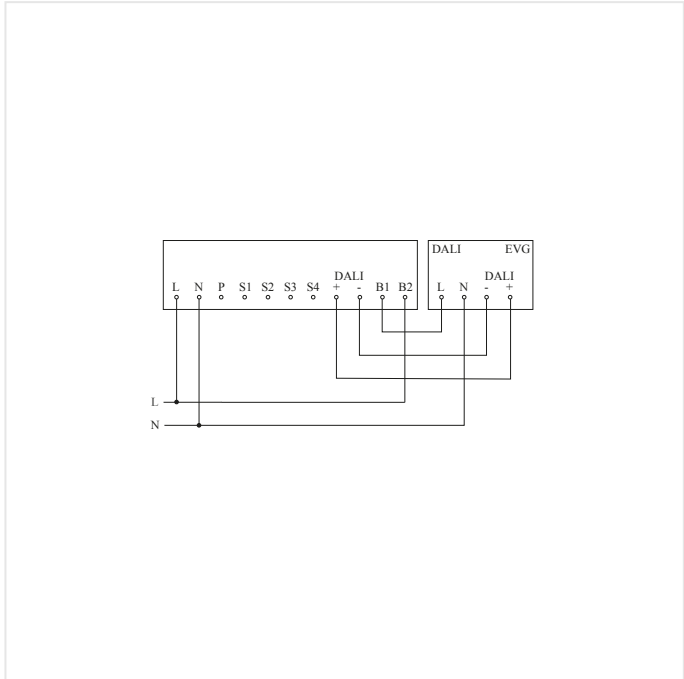
Schema elettrico Master con ballast elettronico OFF
