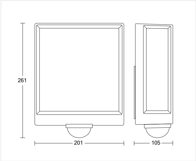
105 x 201 x 261 mm
