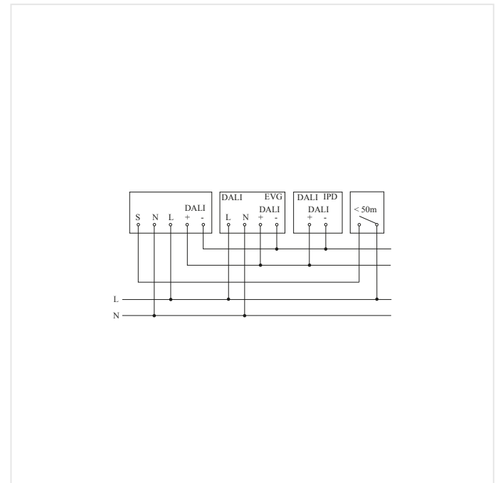
Schaltplan Vernetzung DALI-2 APC mit DALI-2 IPD
